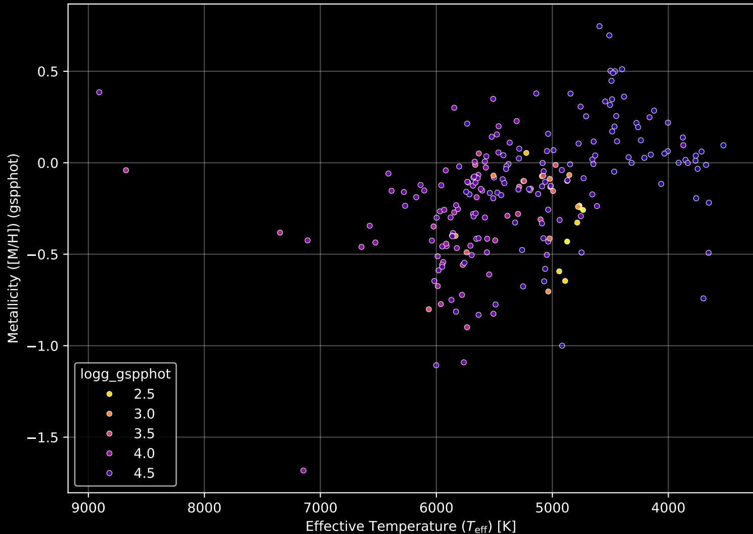
APOGEE DR17 Field: [190-60] Stellar Population Parameters (n= 222)
